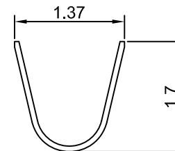
SEC A-A
